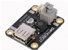
DC DC Step Up Converter 0.9V...5V till 5V 0.6A
