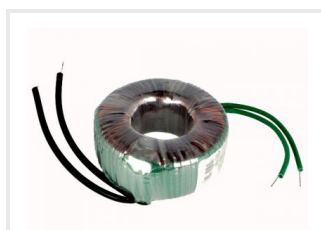
Toroidtransformator 150 VA 230/17 VAC
