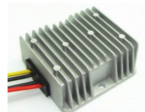
DC/DC stabilisator 24V (9- 32VDC) till 19V, 95Watts max. 5A
