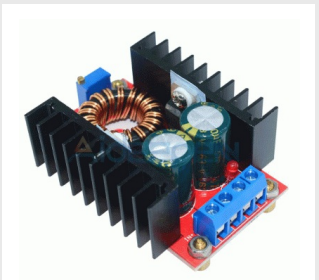
DC-DC Boost Converter Step Up Power Supply Module 10-32V Till 12-35V,
