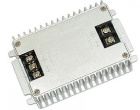
DC/DC Buck omvandlare 12/24V (8...36VDC) till 5VDC 20A
