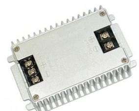
DC/DC-stabilisator 24VDC (8...36VDC) till 12VDC 10A
