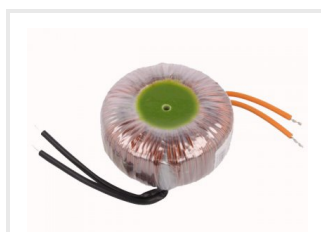
Toroidtransformator 80 VA 230/12 VAC
