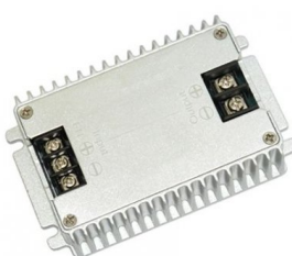
DC/DC-stabilisator 24VDC (8...36VDC) till 12VDC 10A
