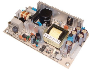
Nättaggregat Mean Well PS- 65-15 15 Volt 65W
