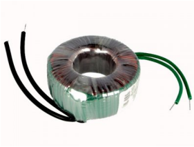
Toroidtransformator 300 VA 230/12 VAC
