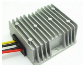
DC/DC Omvandlare 24VDC (17...35) till 19VDC, 190 Watts max. 10A
