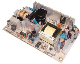
Switchat nättaggregat Mean Well PS-65-7.5 8A
